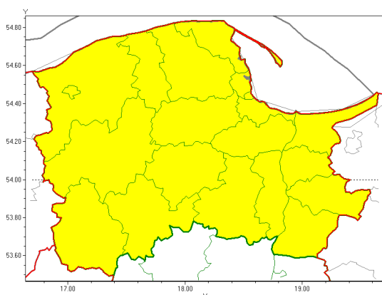
Oblodzenie 2021-04-07 12:21
