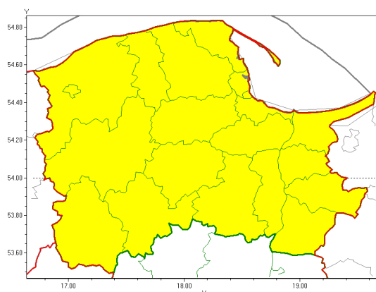
Przymrozki 2021-04-07 12:21
